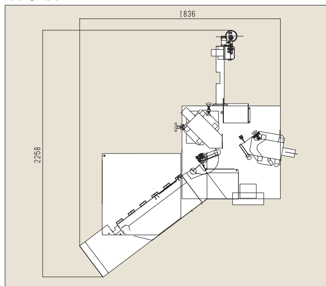
外形寸法図
